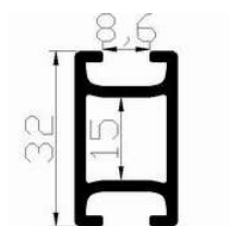
TIG-32 Longitud Max. 6m Perfil travesaño de 32mm
