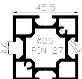
SQ-45,5 Longitud Max. 6m Perfil cuadrado de 45,5mm
