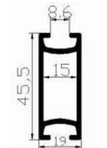
TIG-45,5 Longitud Max. 6m Perfil travesaño de 45,5mm
